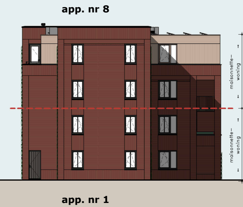
ZIJGEVEL LINKS
