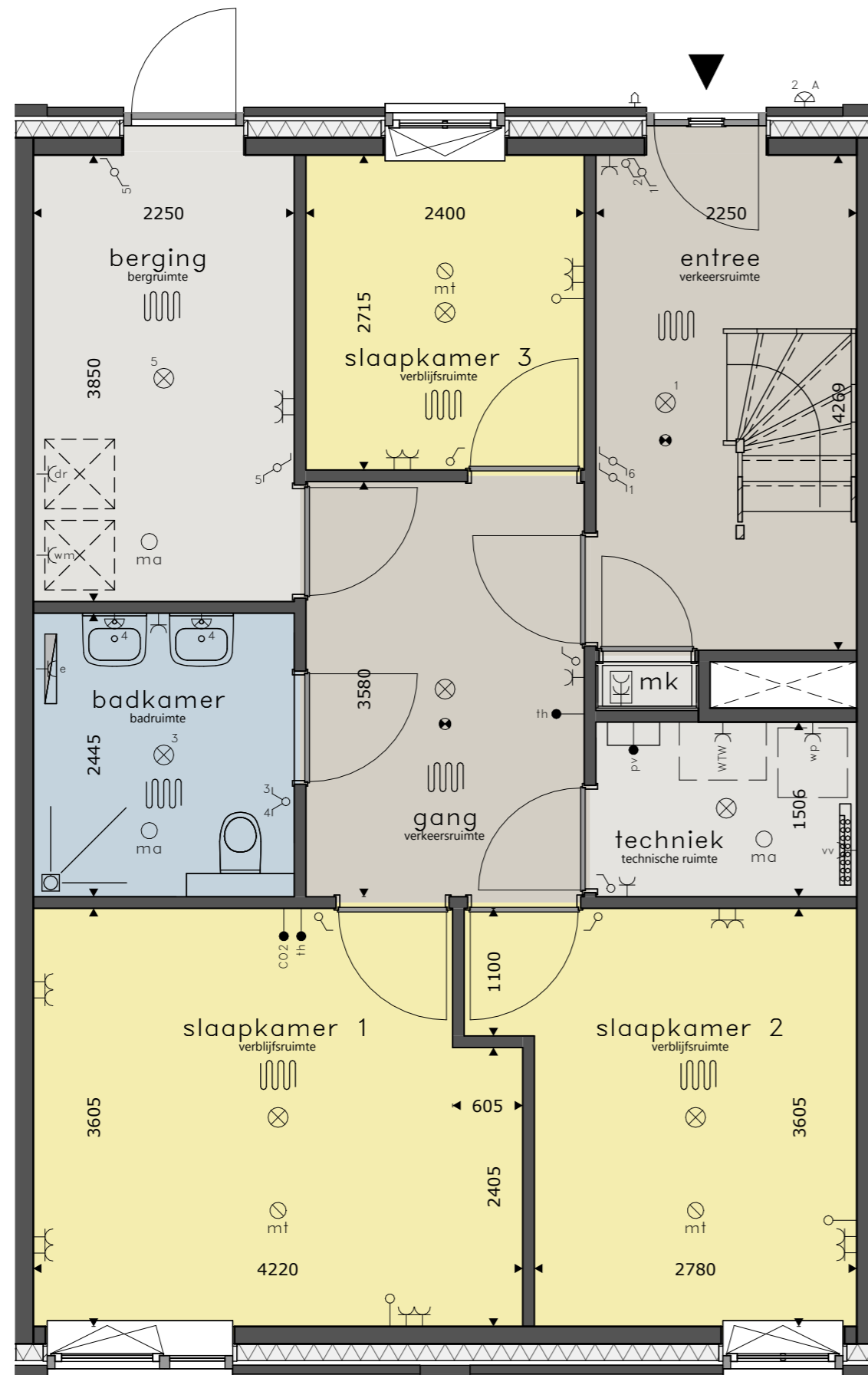
begane grond
